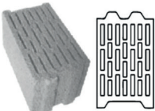
AC BL25 SW YEDİ SIRA BOŞLUKLU BLOK
