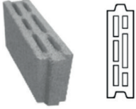
AC BL10 SW İKİ SIRA BOŞLUKLU BLOK
