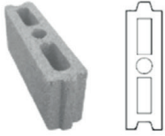
AC BL10 G TEK SIRA BOŞLUKLU BLOK
