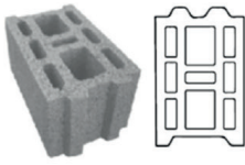
AC BL25G ÜÇ SIRA BOŞLUKLU BLOK
