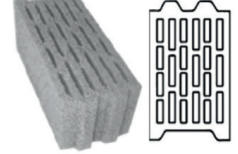
AC BL19 SW ALTI SIRA BOŞLUKLU BLOK
