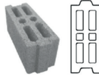
AC BL15 G İKİ SIRA BOŞLUKLU BLOK
